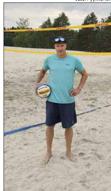
Jussi Pyykkönen
